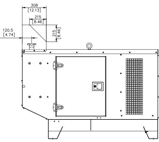
OPTION: CAPOT INTERIEUR / INSIDE CANOPY
